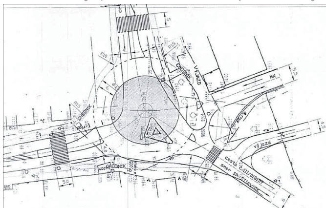
Návrh riešenia križovatky ciest pri pomníku padlých.
